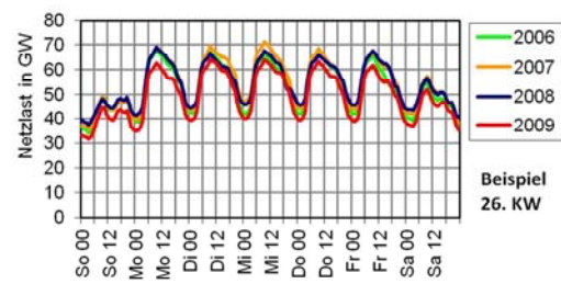
tageszeitliche Netzlasten in Deutschland
