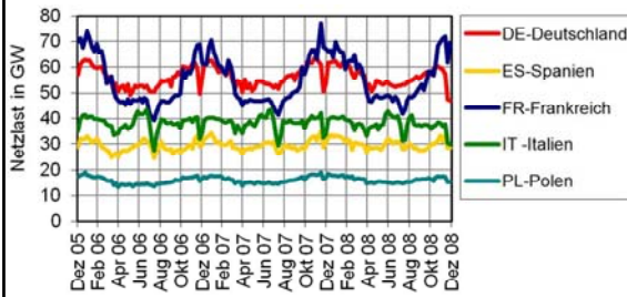
wöchentliche Netzlasten europäischer Länder
